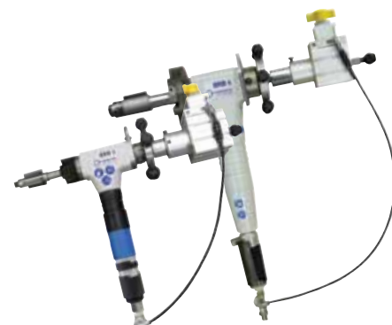
par ex. BRB 2 et BRB 4 Air comprimé/Auto avec système de serrage "NC"
